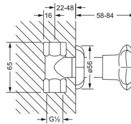
mit Einbaukörper 1/2"
