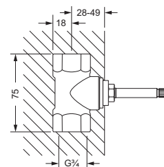
Einbaukörper 3/4"
