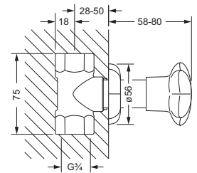
mit Einbaukörper 3/4"
