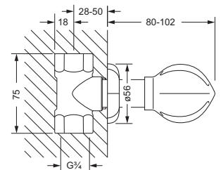
mit Einbaukörper 3/4"
